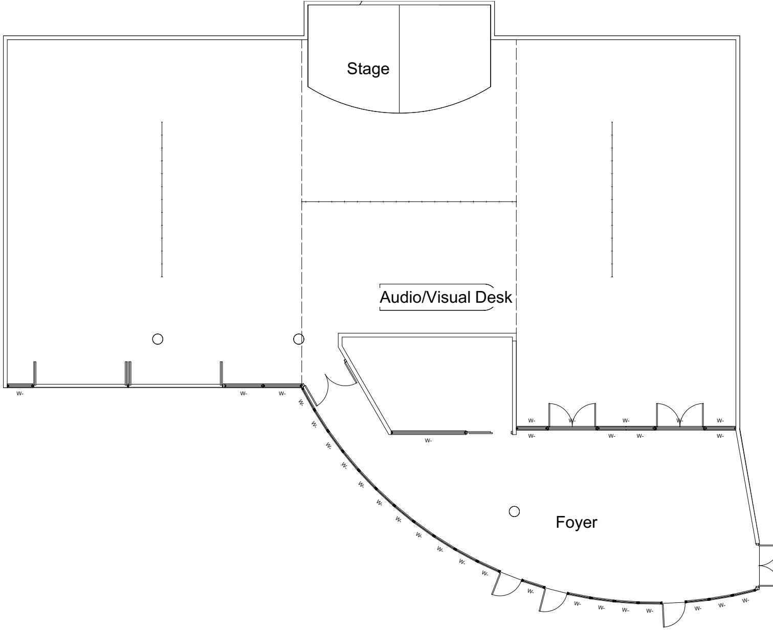
1 Glasshouse Scale: 1:150
